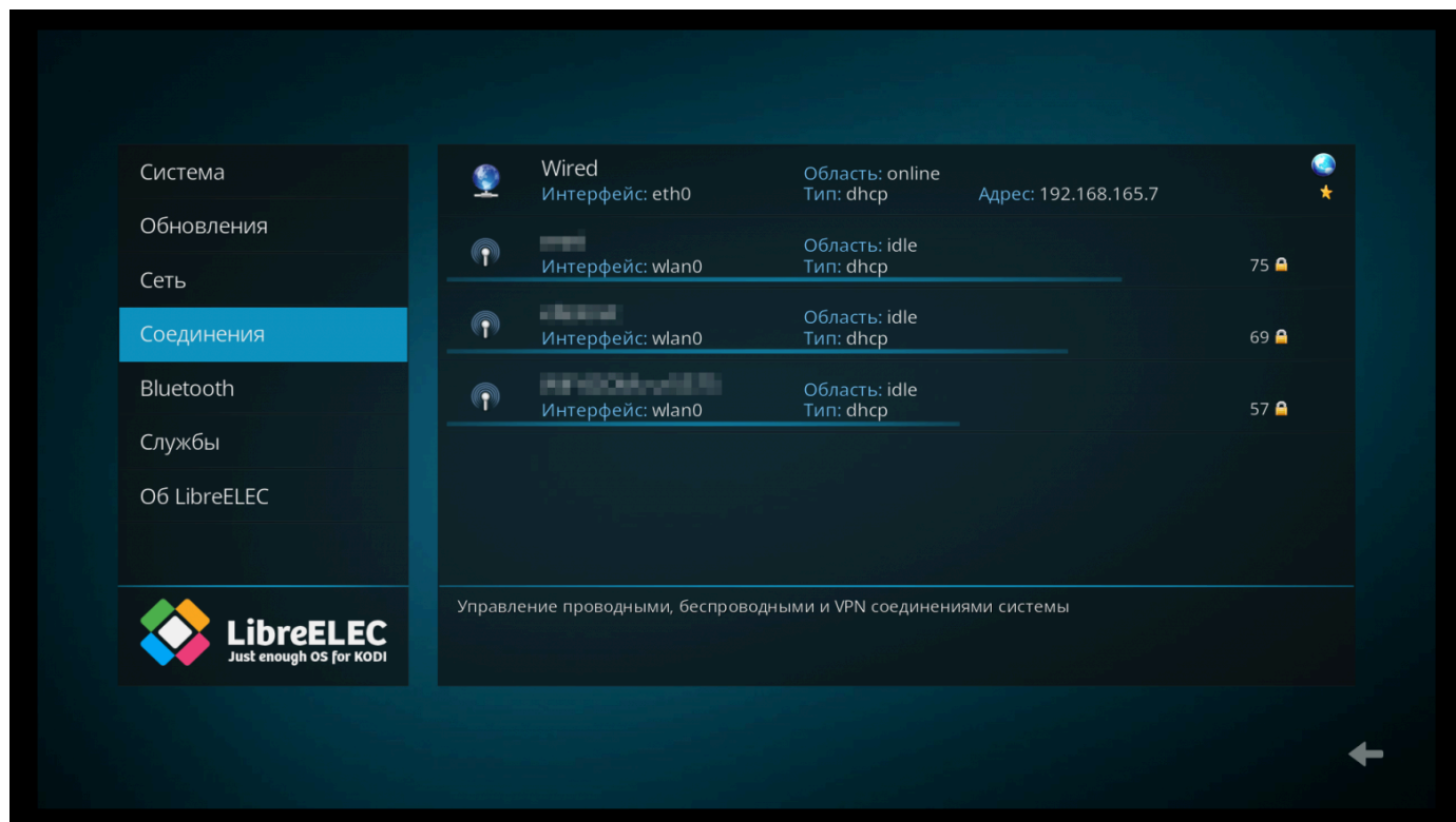
Вкладка Соединения
