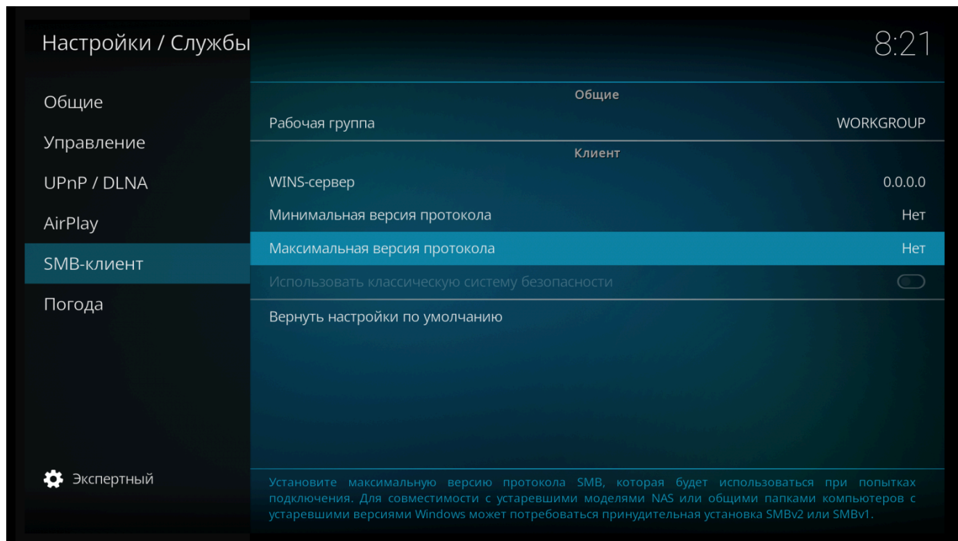
Настройки Samba
